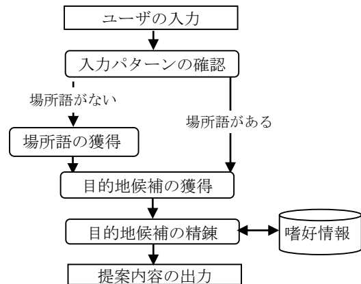
図 1. 旅行提案システム概要図
