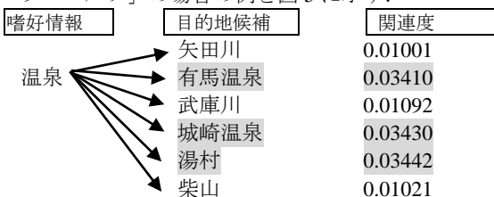
図 5. 目的地候補の精練
