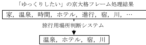
図 2. 場所語の獲得 1
