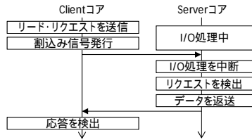
図4 割込み方式概要
