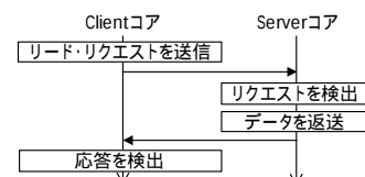
図2 専用コア方式概要
