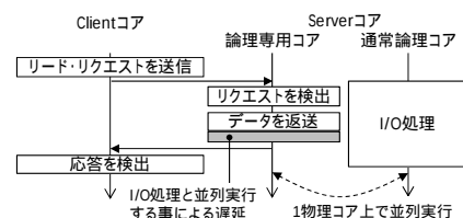
図3 論理専用コア方式概要
