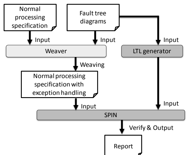
図 1 提案手法
