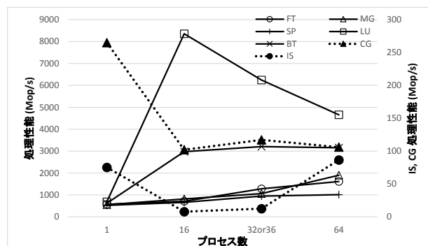
図 3 並列処理性能
