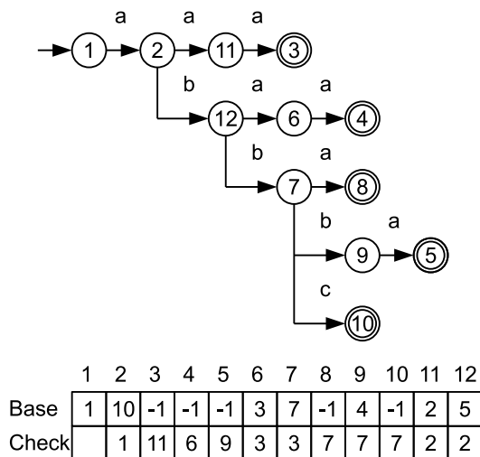
図 2: キー集合 K を表現するトライ図とダブル配列 1
