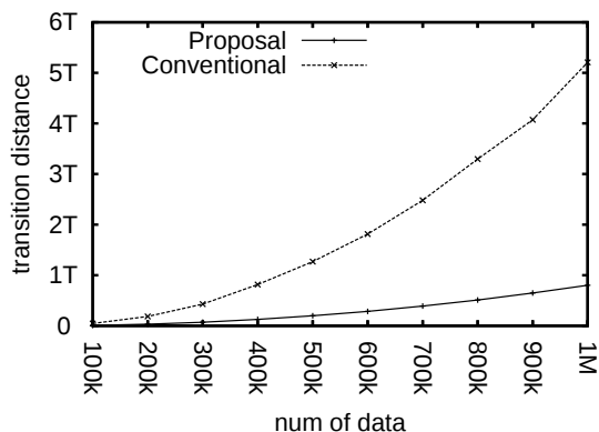
図 16: 変換前後の遷移距離総和
