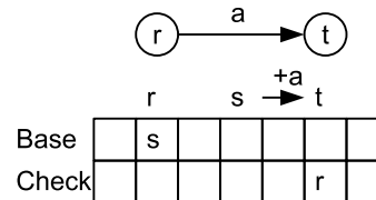
図 1: 節点間の遷移
