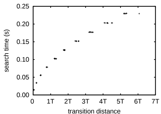
図 17: 遷移距離と探索時間の散布図
