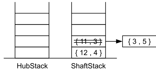
図 9: Sieve({3,5}) 後のスタック
