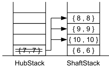
図 11: Locate({7,7}) 後のスタック
