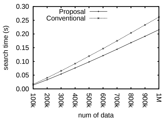
図 15: 変換前後の探索時間
