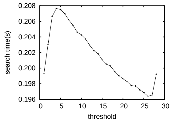
図 13: \theta を変動させた際の探索時間
