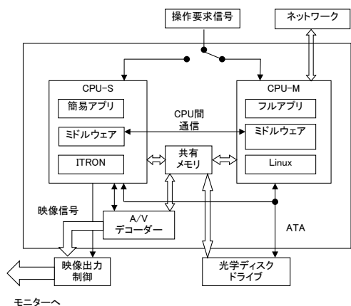
図4. BDプレーヤーシステム
