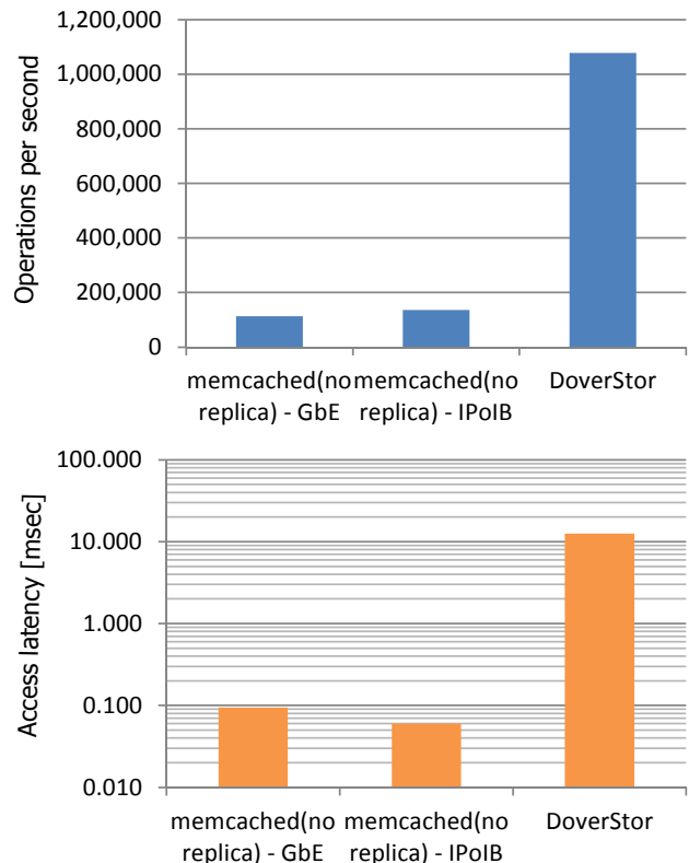
図 4: 既存技術との比較
