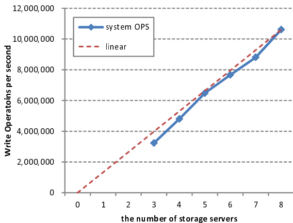
図 5: ストレージノード台数と OPS 性能の関係
