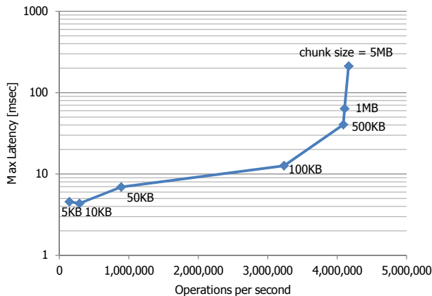
図 3: 一括処理要求数を変化させたときの最大レイテンシと OPS 性能の関係（ノード 3 台構成）
