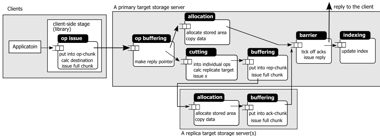
図 2: Staged ストレージ設計による Write 要求のデータフローおよび制御フロー
