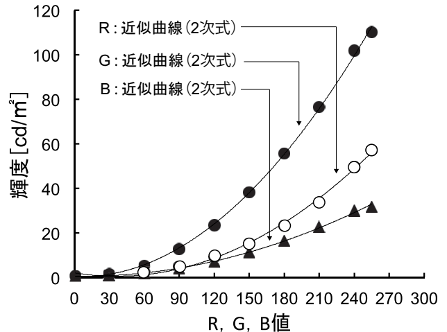
図2: 画面の色と輝度の関係 (バックライト最大時)
