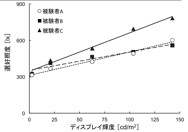
図 5: 画面の色と輝度の関係 (バックライト最大時)
