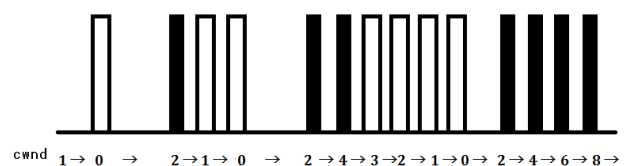
図2.2 パケットフローとその輻輳ウィンドウの推移
