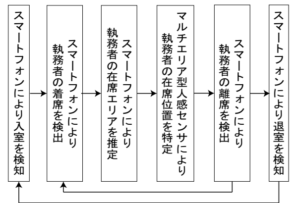
図 1: 在席・離席検出手法に用いるアルゴリズム
