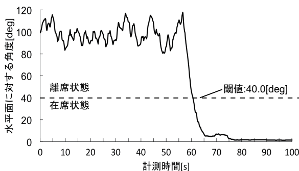
図 3: スマートフォン端末の水平面に対する角度計測
