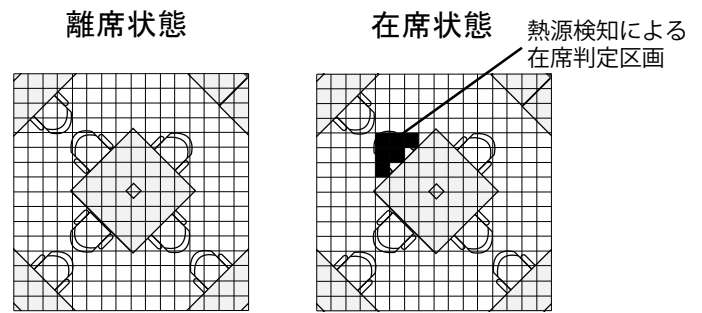
図 4: マルチエリア型人感センサによる在席検出
