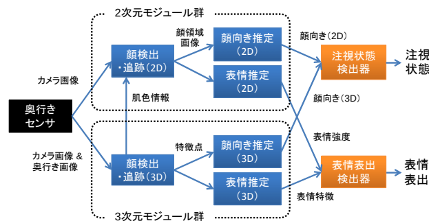
図 1 視聴状況推定の流れ
