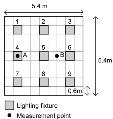
図 2 実験環境および実験器具の配置
