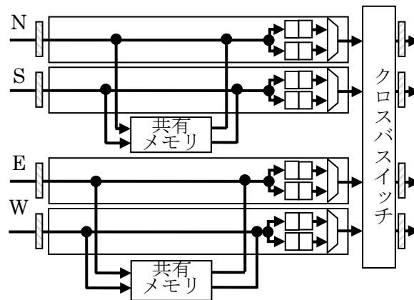
図 5. 2リンク共有のルータ構造
