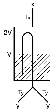
図 6: 1-tube 方式の COPY 回路
