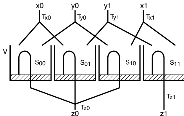
図 11: 2-tube 方式の AND 回路
