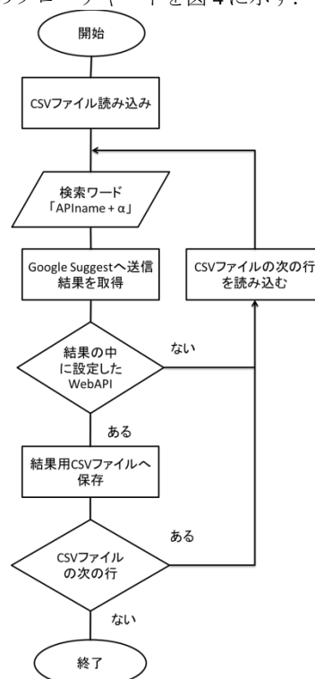
図4 Google Suggest へのクエリ送信時のフローチャート
