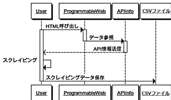
図3 ProgrammableWeb に対するスクレイピングのシーケンス
