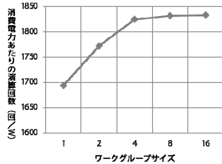
図7 ワークグループサイズに対する消費電力あたりの演算回数
