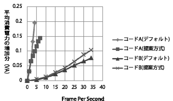
図 5 データ入力速度に対する平均消費電力
