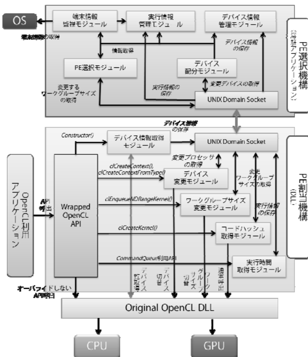
図3 提案方式のモジュール構成
