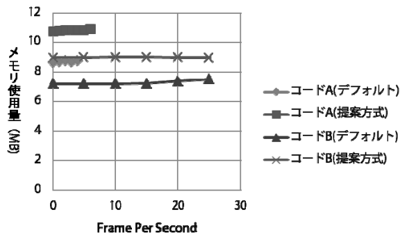
図6 データ入力速度に対するメモリ使用量
