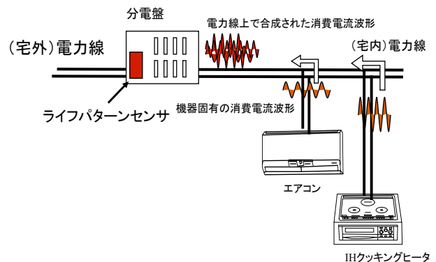
図.1 ライフパターンセンサの概要
