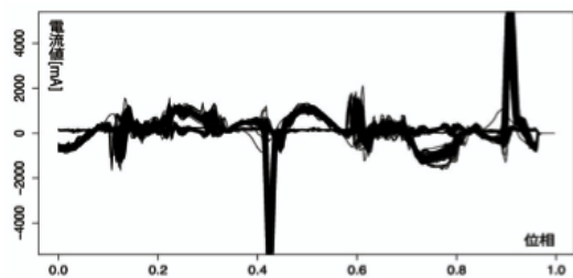
図.11 電子レンジ単体動作時の消費電流波形
