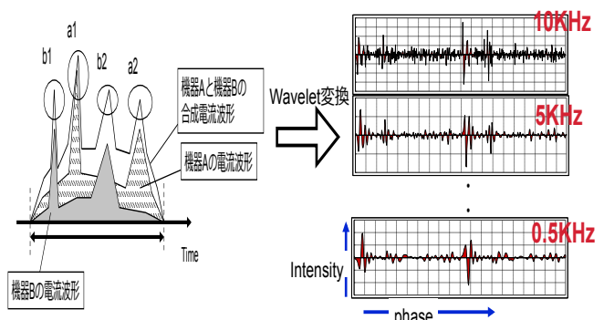
図.2 ライフパターンセンサの動作原理
