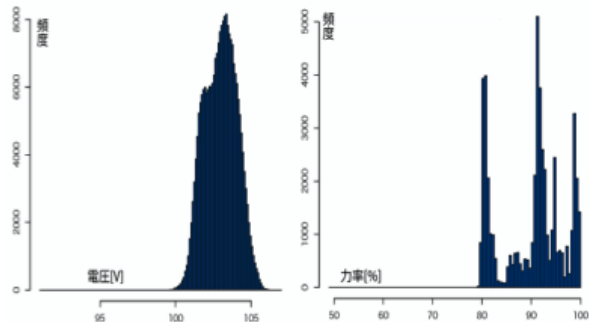
図.9 電圧・力率の変動の分布
