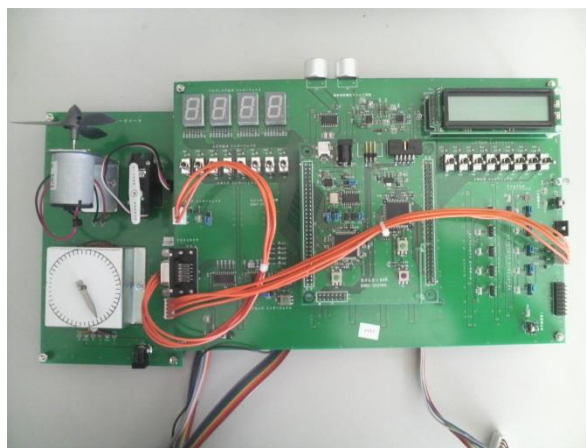
図 2.1.1.1 カメレオン AVR・カメレオン AVR 指南 (右) とオプションボード (左)
