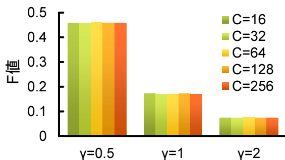
図 3: サポートベクターマシンによる予測を検証用データセットに適用したときの F 値. C と \gamma はサポートベクターマシンのパラメータである.
