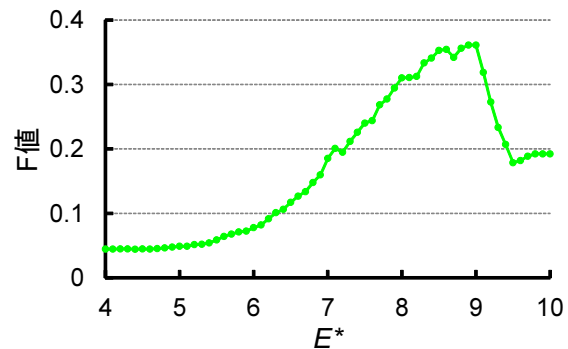
図 4: ZDOCK による予測を構造データセットに適用したときの F 値.
