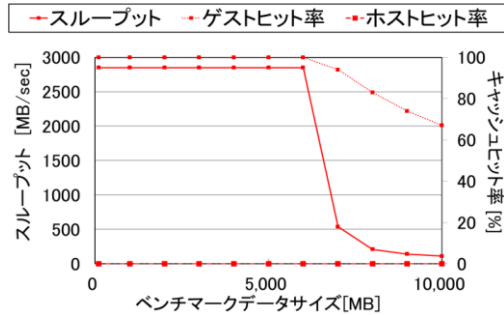
図 4 ゲスト OS メモリ 7000MB, ホスト OS メモリ 1000MB におけるキャッシュヒット率と I/O 性能
