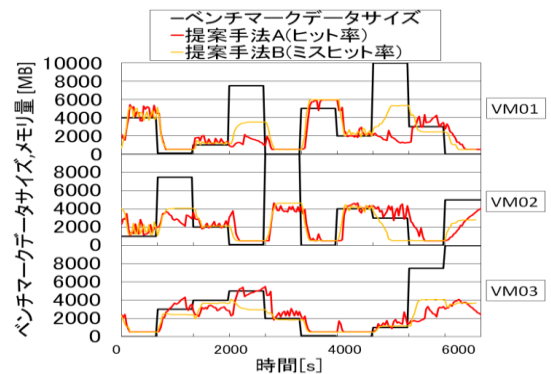
図 7 VM メモリ量変化の推移
