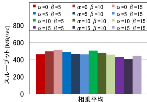
図 9 提案手法の分配量変更による比較 (相乗平均)
