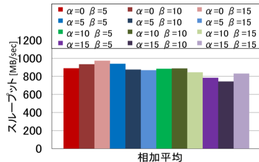
図 8 提案手法の分配量変更による比較 (相加平均)
