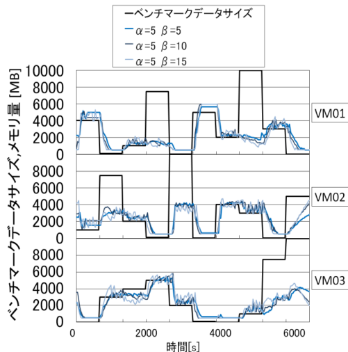
図11 VMメモリ量変化の推移（分配量変更 \alpha=10 ）
