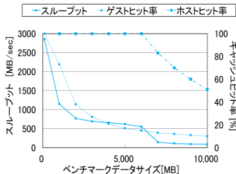
図 5 ゲスト OS メモリ 1000MB, ホスト OS メモリ 7000MB におけるキャッシュヒット率と I/O 性能
