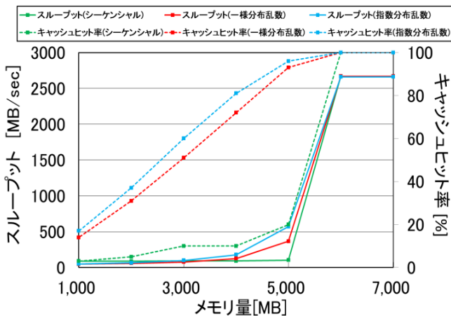
図 2 キャッシュヒット率とスループットの測定
