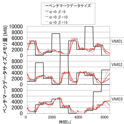
図10 VMメモリ量変化の推移（分配量変更 \alpha=0 ）
