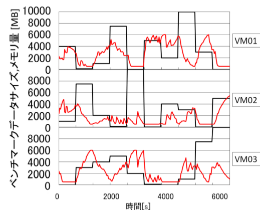
図 15 VM メモリ量変化の推移
