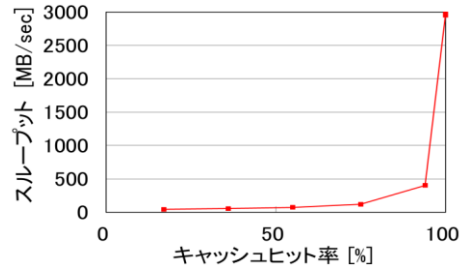
図 3 キャッシュヒット率とスループットの関係
