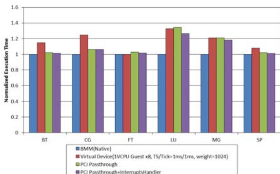
図 9 NPB3.3.1-MPI クラス C 8 ノード 64 プロセスの実行結果
