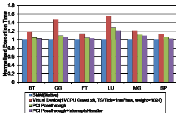
図 8 NPB3.3.1-MPI クラス B 8 ノード 64 プロセスの実行結果
