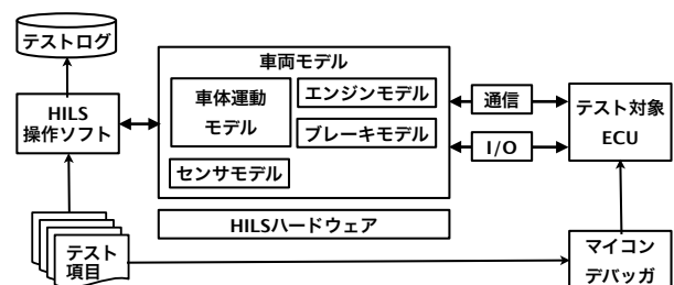
図 1: HILS 環境の構成
