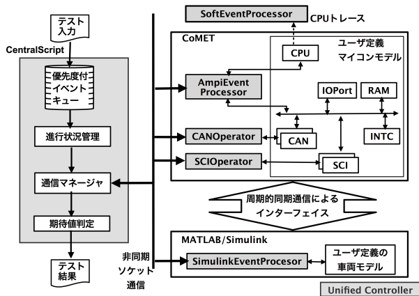
図 5: UC を導入した vHILS の構成
