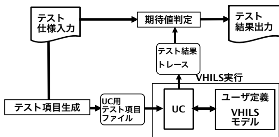
図 6: vHILS 自動実行システムの運用形態
