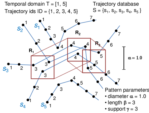
図 1 例: 軌跡データベース S_1 である. ID = \{1, \dots, 5\} と T = [1, 7] と (1.0, 2, 2) -フログパターン P_1 = (X_1, I_1) = (\{2, 3, 4\}, [3, 5]) になる. 幅 \|P_1\|_\infty^{S_1} \leq 1.0 , 長さ len(P_1) = 3 と支持度 supp(P_1) = 3 . ここで線は軌跡データに代表している. 点の隣の数字は時間印である.
