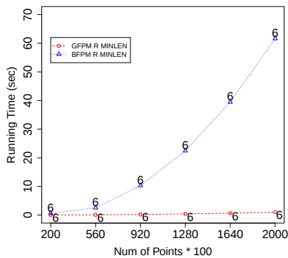
図6 実験 1b: RFPM (RFPM R) と G-RFPM (GFPM R) の計算時間とボタン数である。
