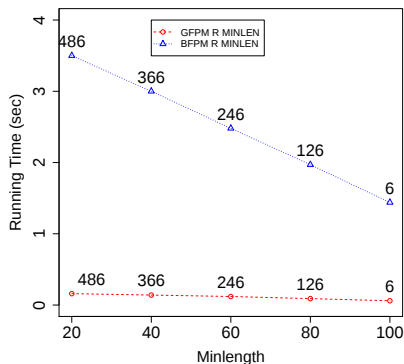
図8 実験 3b: RFPM (RFPM R) と G-RFPM (GFPM R) の計算時間とボタン数である。
