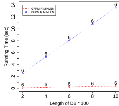
図7 実験 2b: RFPM (RFPM R) と G-RFPM (GFPM R) の計算時間とボタン数である。
