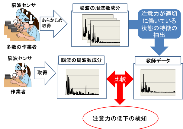
図 1: 手法概要図
