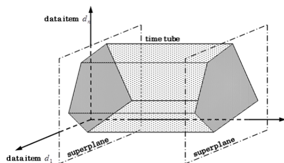
図 5: TimeTube
