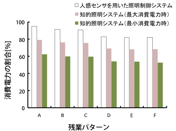
図3 残業パターン別平均消費電力
