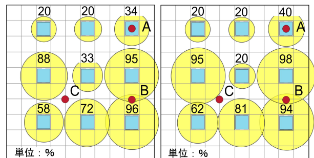
(1) スマートフォンを用いた場合 (2) 照度センサを用いた場合 図4 各照明の点灯パターンの比較（設定1）
