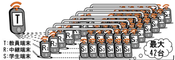
図 1. 本システムのツリー型ネットワーク
