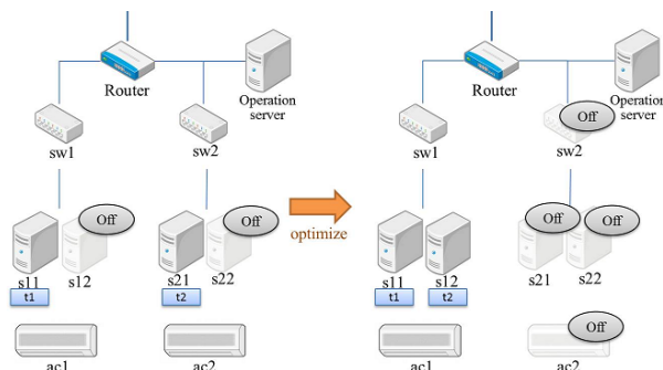
図 3: ネットワークシステムにおけるプランニングの例
