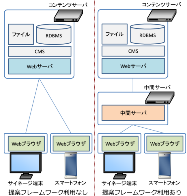
図3 検証用システムのシステム構成図
