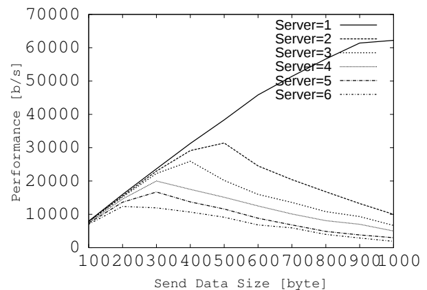
図 3: 受信端末数と通信性能の関係
