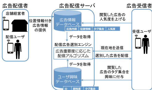
図3 本提案システムのモデル
