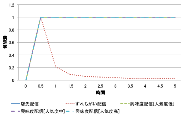
図 12 各モデルのステップごとの興味度 1 のときの満足率
