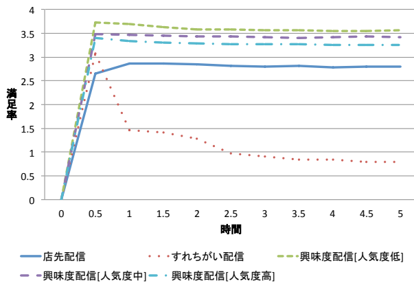
図 11 各モデルのステップごとの歩行者満足率
