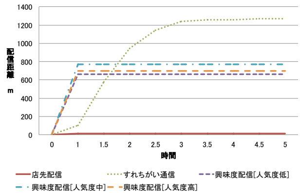
図10 各モデルのステップごとの広告配信最大範囲
