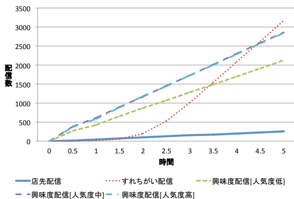
図9 各モデルのステップごとの広告配信数
