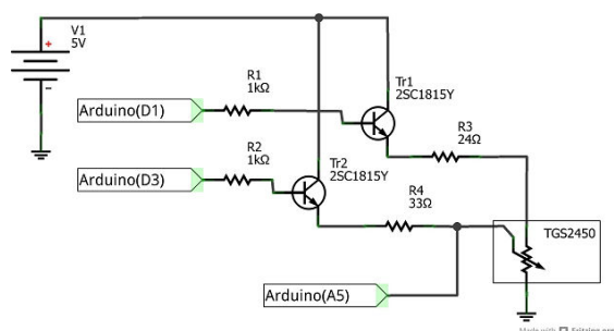
図 1: 臭気センサの回路図
