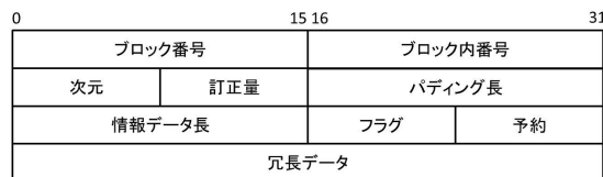
図 8: RS ヘッダのフォーマット
