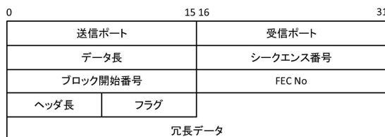
図 4: 共通ヘッダのフォーマット
