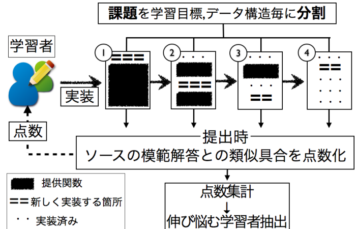
図 1: 手法の全体図
