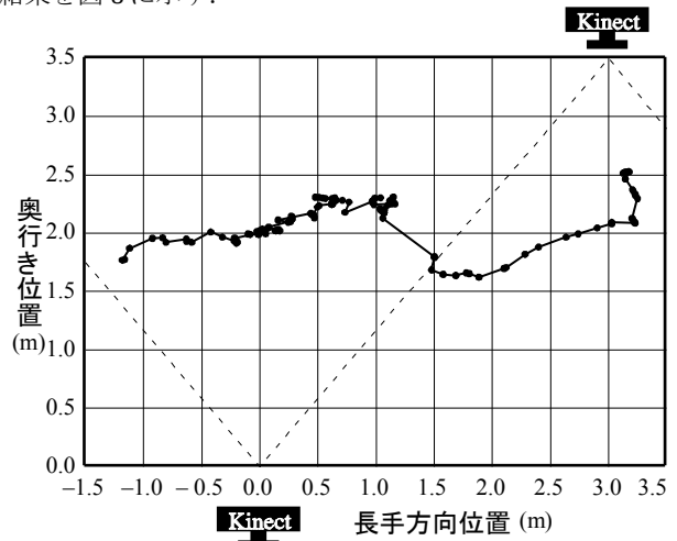
図 8 サーバ側で扱った人物位置情報の軌跡
