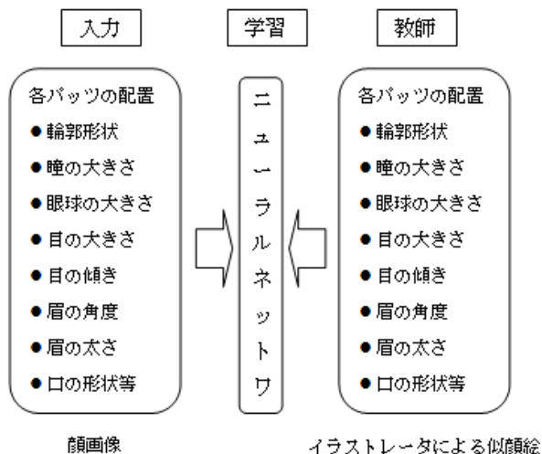
図4 似顔絵の学習
