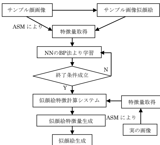
図1 似顔絵生成の流れ
