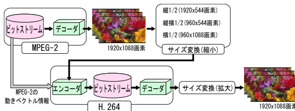
図 2: 提案手法の処理手順
