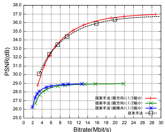
図7: Crowded CrosswalkにおけるRD特性の比較
