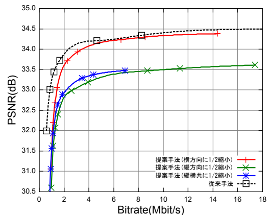
図6: Flower BasketにおけるRD特性の比較
