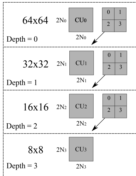
図 1: Coding Unit の階層構造
