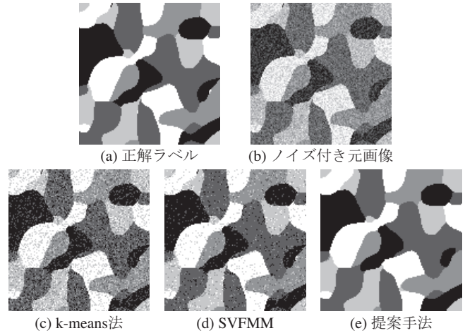
図 1 C = 5, \sigma_N = 0.10 における元画像と分割結果の一例
