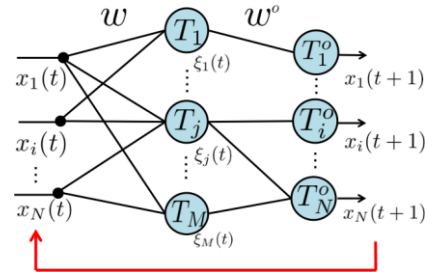
図 1 DBNN モデル
