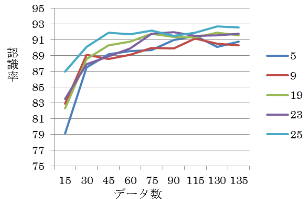
図 3 iris データの認識率
