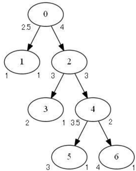
図 1 SGNT の生成例
