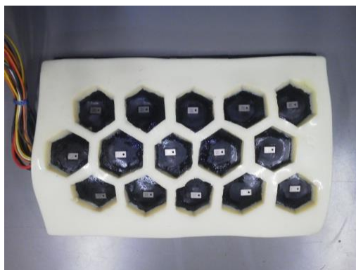
図1 マルチチャンネルセンサ
