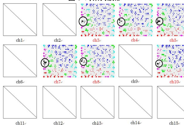
図 4 SOM 結果
