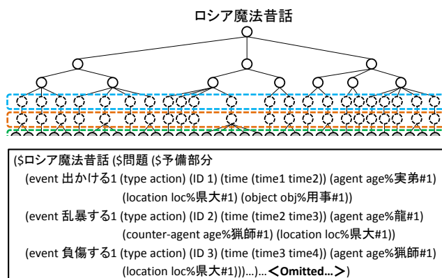
図4 プロップに基づくストーリーグラマーから生成される物語の構造
