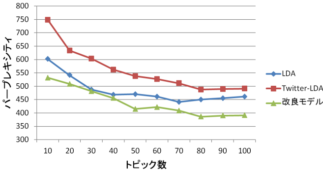
図 2: パープレキシティの比較
