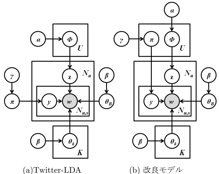
図 1: グラフィカルモデル
