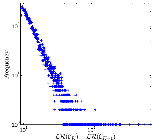
図 1: \mathcal{LR}(C_k) - \mathcal{LR}(C_{k-1}) の度数分布
