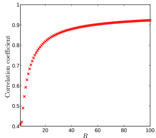
図 2: A_u と u のレビュー投稿数の相関係数の推移
