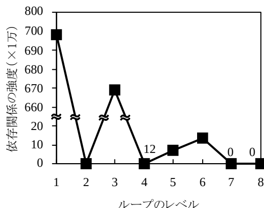
図 3 依存関係の強度 (433.milc)
