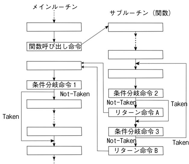
図3 命令実行の流れ（例2）
