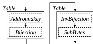
図 4 AddroundKey と SubBytes のテーブル置換
