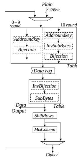
図 5 WhiteBox_by_BlockRAM 回路
