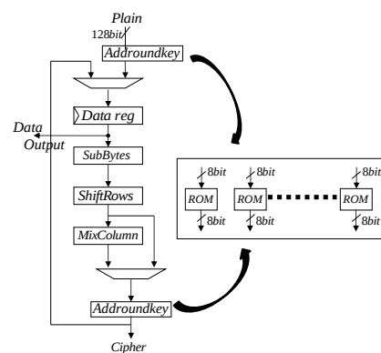
図 3 xor_by_ROM 回路
