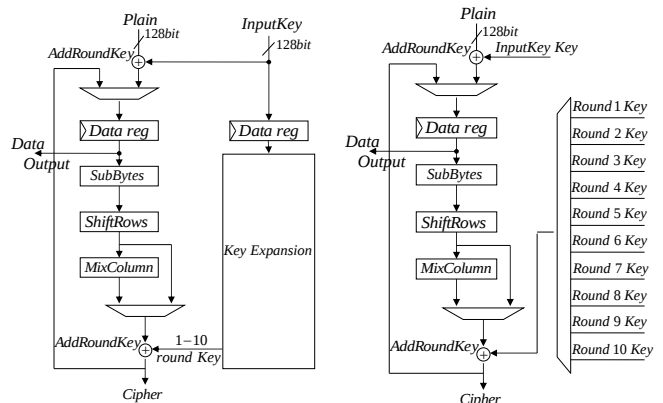
図 1 AES 暗号化回路
