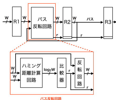
図 1: バス反転回路
