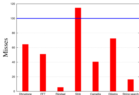
図 2：提案手法のミス数
